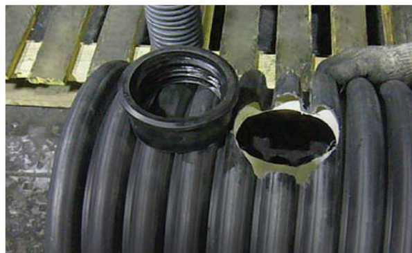
2. Подготовить манжету для помещения в отверстие.
