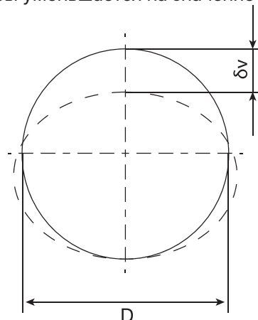
Рисунок 4. Деформация трубы от вертикальной нагрузки.
