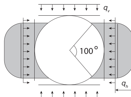
Рисунок 5. Модель распределения давления грунта по скандинавской методике
