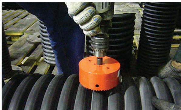
1. В шахте колодца вырезать отверстие с помощью фрезы.
