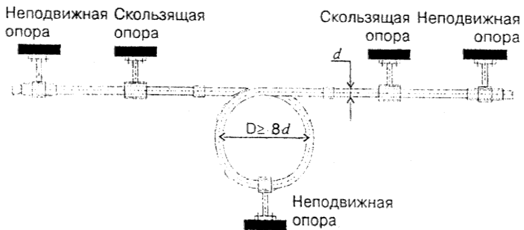
Рис. 2.6. Петлеобразный компенсатор
