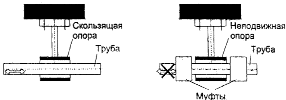
Рис. 4.1. Виды опор
