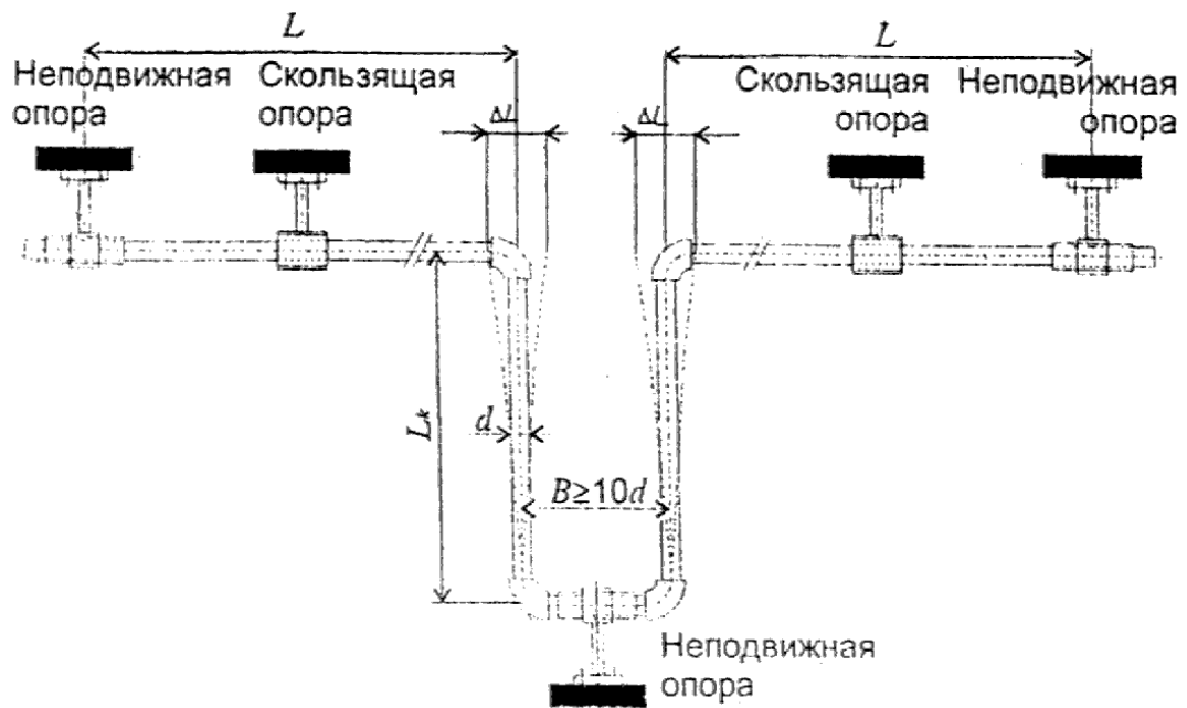
Рис. 2.5. П-образный компенсатор
